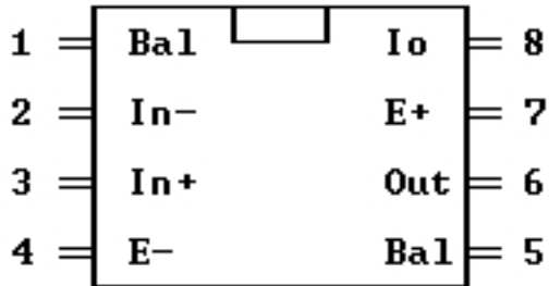
КР140УД1208
