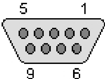
9-контактный D-SUB разъем
